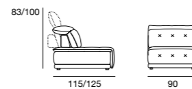
Elemento 1 posto_1 seater element
